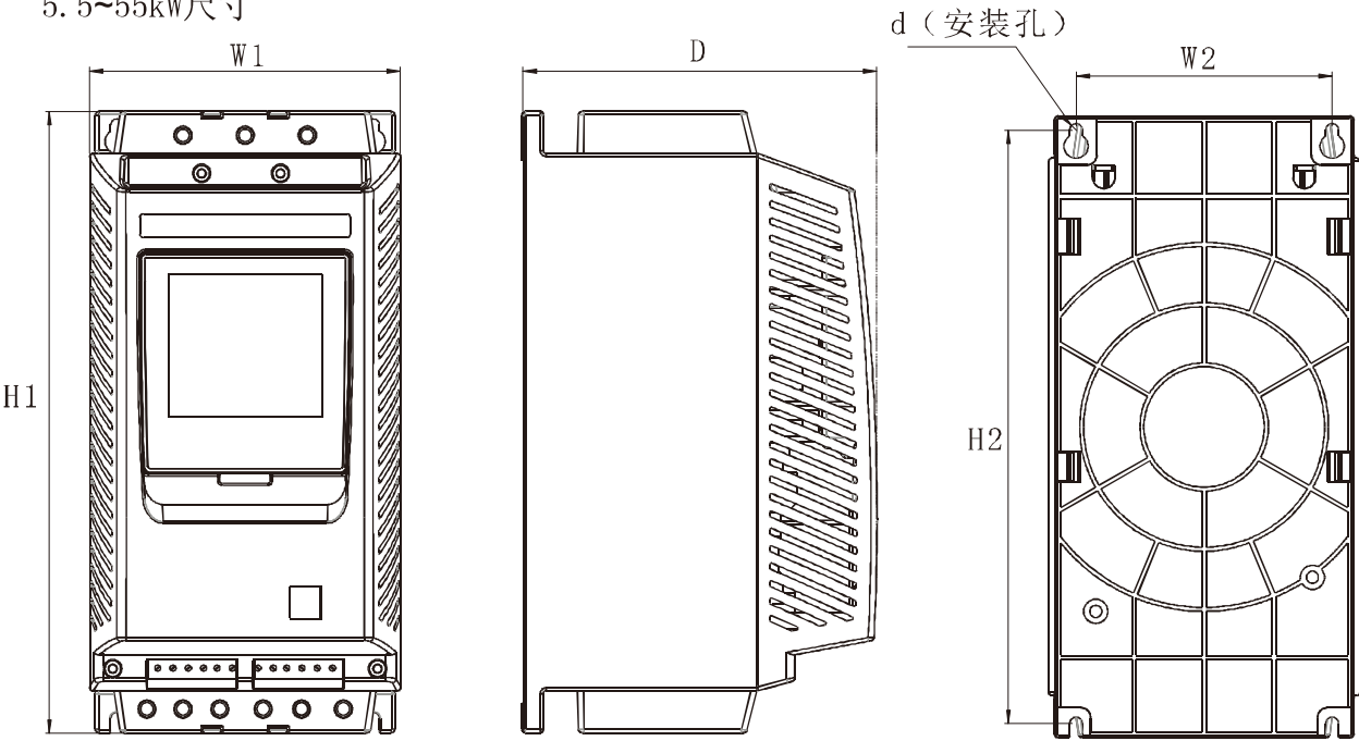
KNRG-2000 外置旁路型5. 5KW~ 55KW软起器外形及安装尺寸见表：
